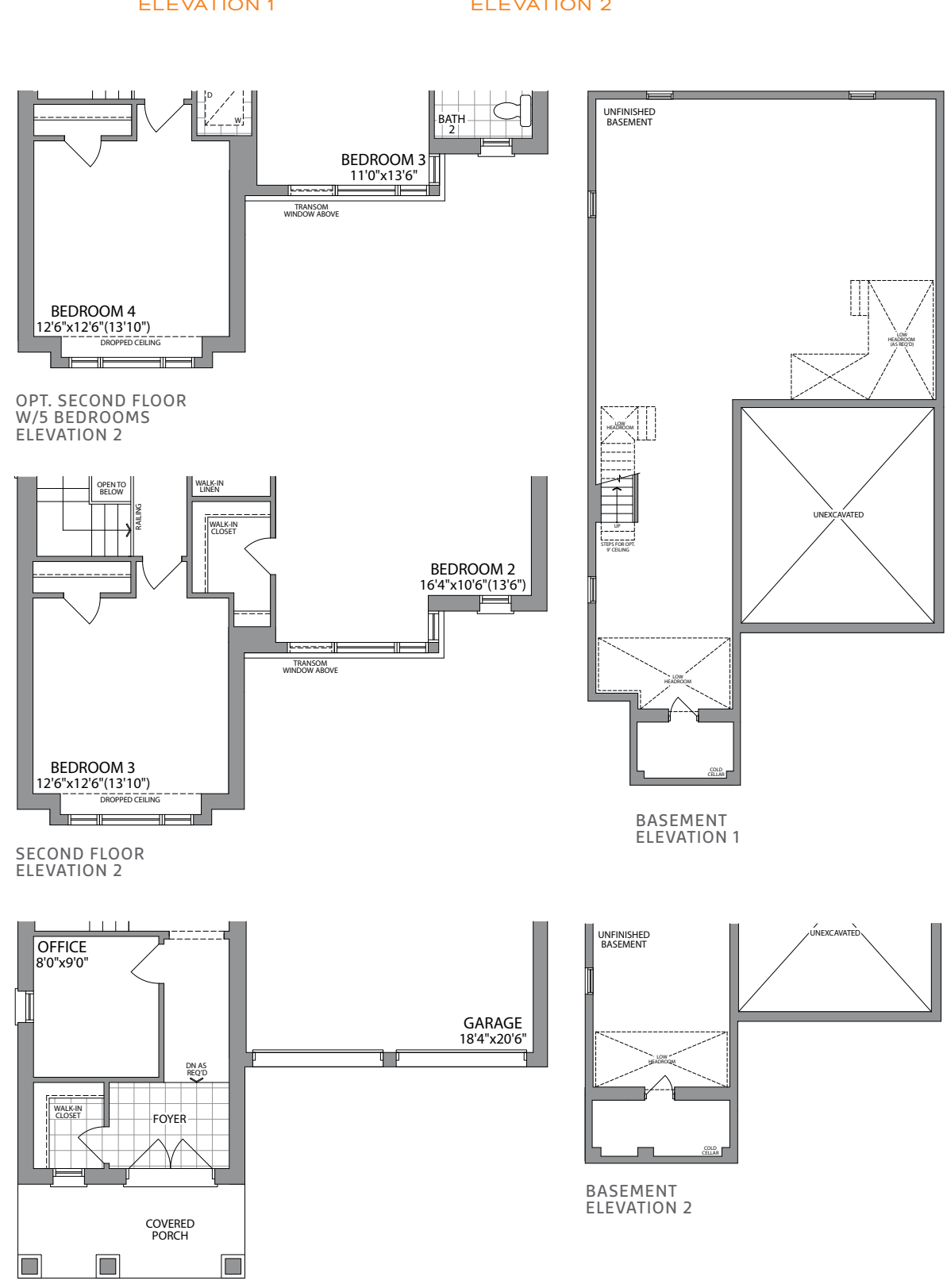
ELEVATION 1
